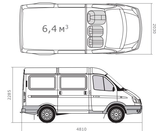
ГАЗ-2752 «СОБОЛЬ»
