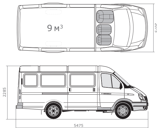
ГАЗ-2752 «СОБОЛЬ»
