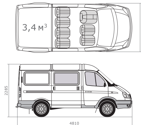
ГАЗ-2752 комби «СОБОЛЬ»
